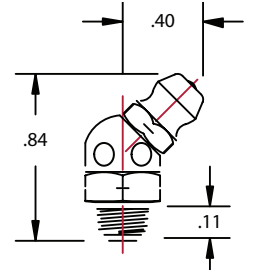
1/4"-28 TAPER THD. (SAE-LT)
